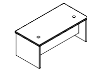
ER21 主管桌 1800(W)×900(D)×760(H) 1600(W)×800(D)×760(H)
